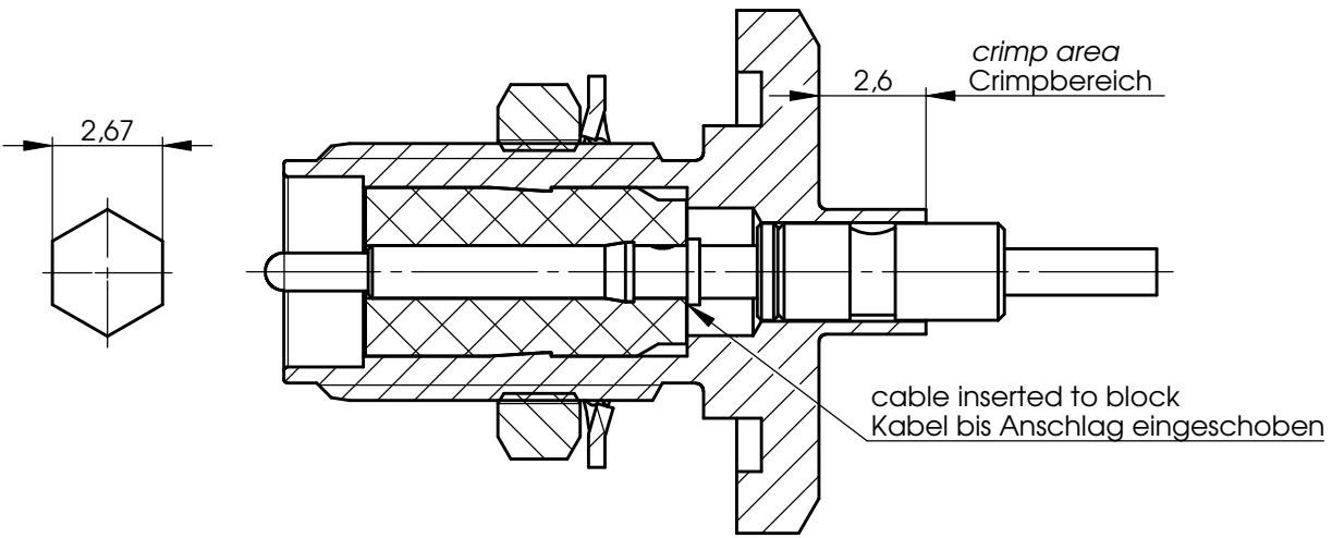
crimp insert / Crimpeinsatz: N01001A0010
